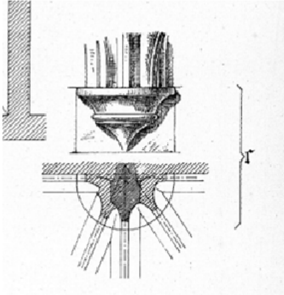
Abbildung 98: Gaming, ehemalige Kartause, Architekturzeichnung der Wiener Bauhütte, Nr. 49, Victor Lunz, 1866, Grundriss der Kirche, Detail der Wandkonsole in der Nordkapelle.
